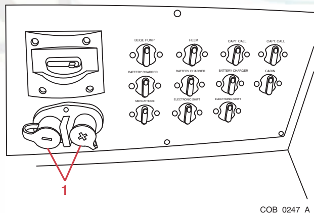
1 – Receptacle
